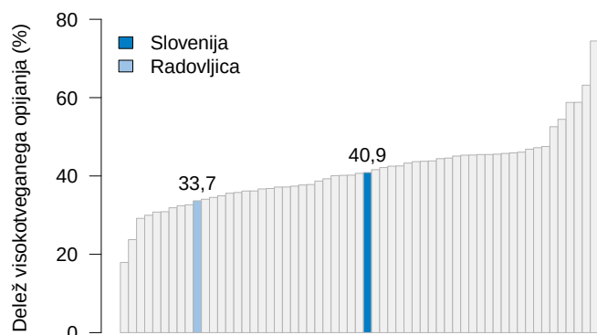
Slika 5: Delež oseb, starih 15 let in več, ki so se v zadnjem letu visokotvegano opile; upravna enota Radovljica, v katero spada občina Bled, 2014.
